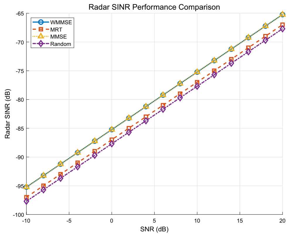
Fig. 4 Radar SINR versus SNR
